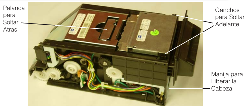
JCM " WBA " El Montaje del Validador solo Acepta un Billete
